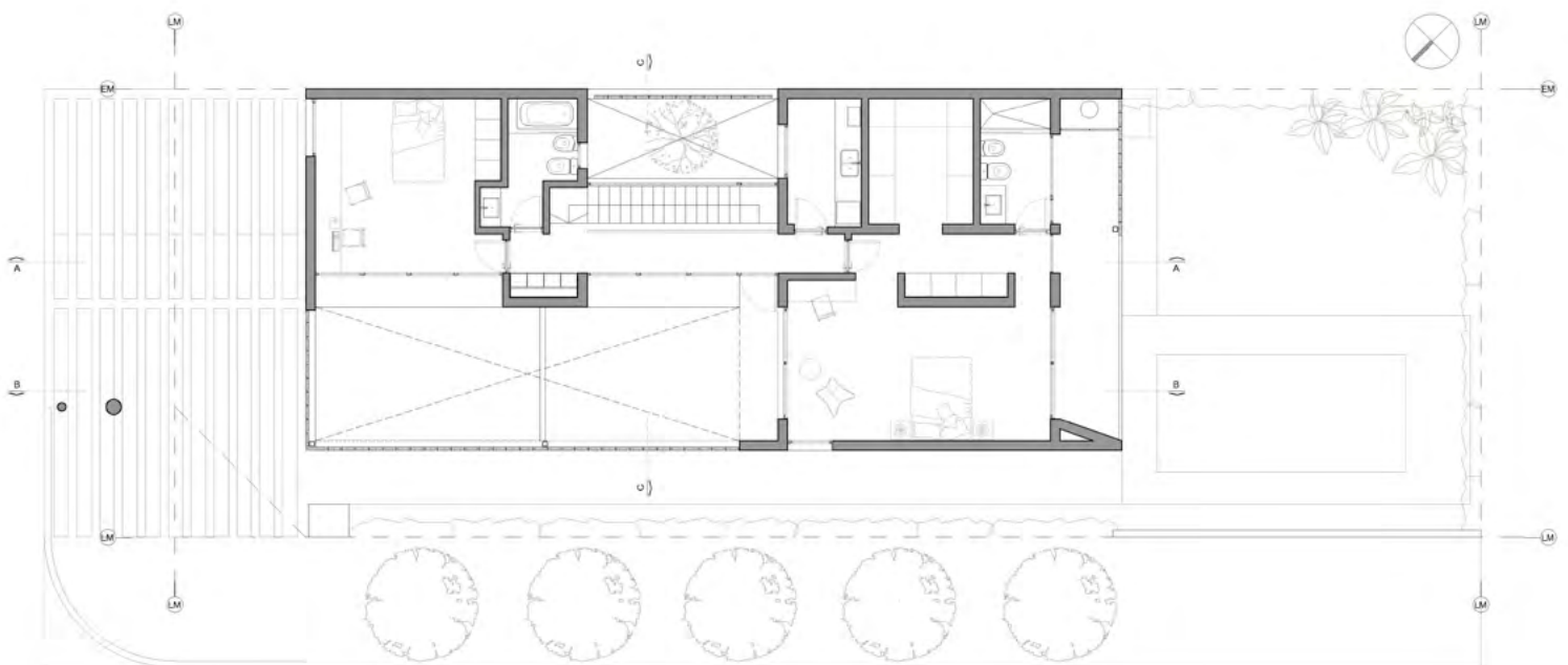
PLANTA ALTA 0 1 2 3
