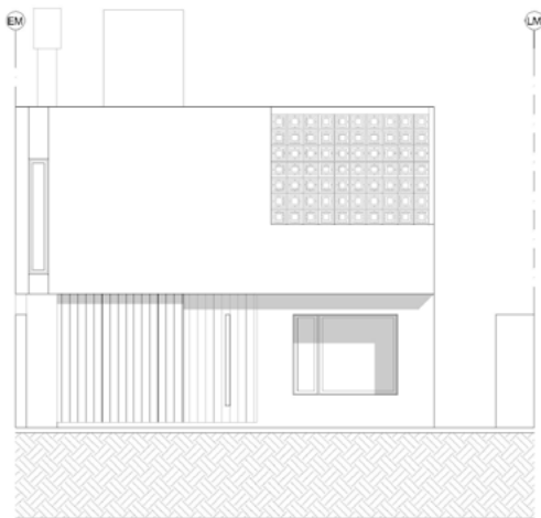
FACHADA FRENTE
