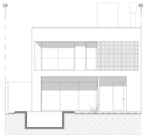
FACHADA CONTRAFRENTE
