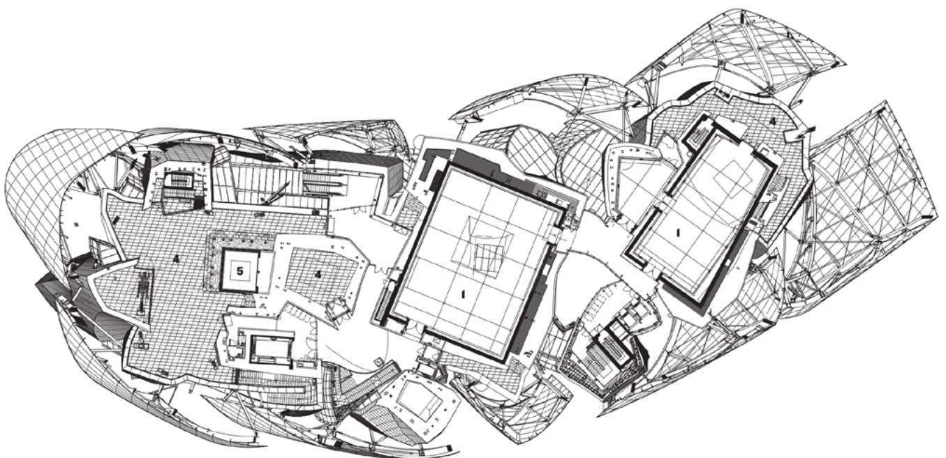
PRIMER PISO
