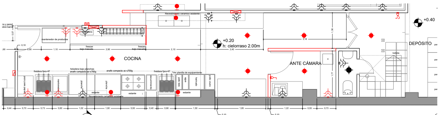
ELEVACIÓN COCINA - ESC. 1:50
