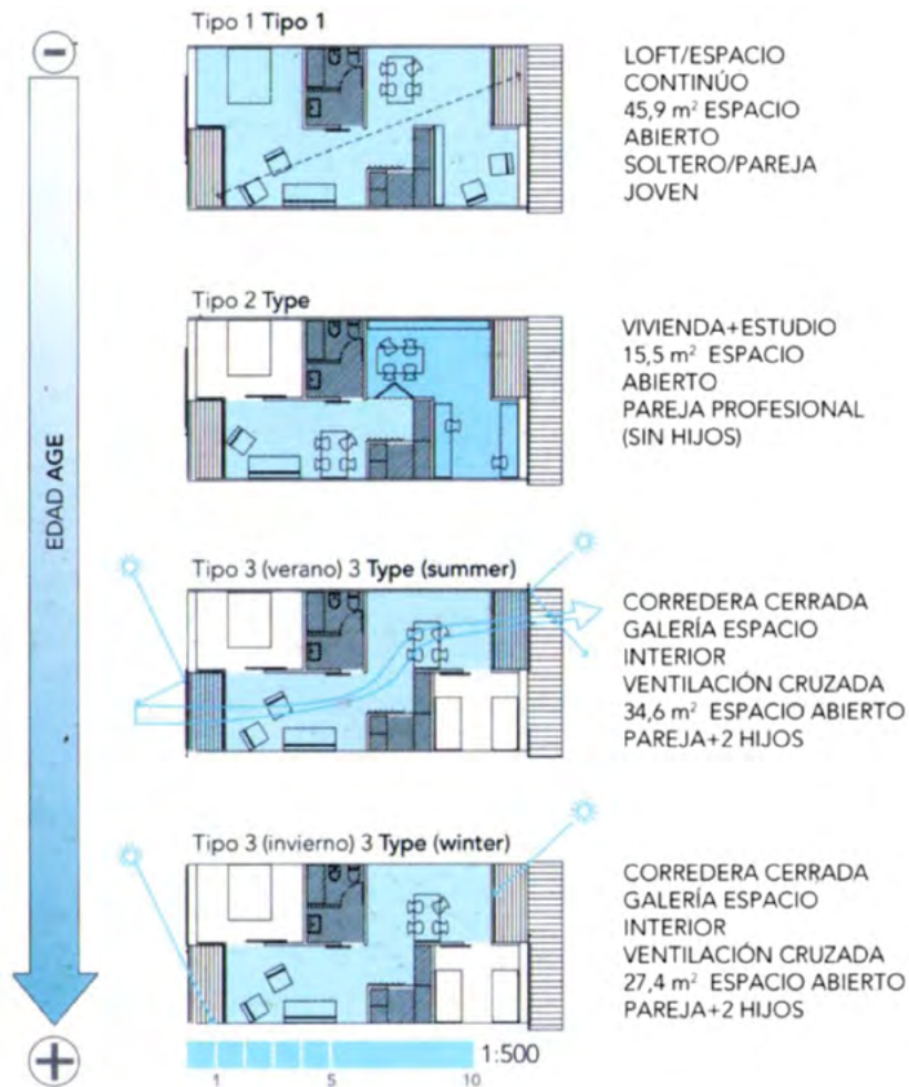
PLANTA EVOLUTIVA. VIVIENDAS EM PARDINES, COLL-LECLERC, 2005
