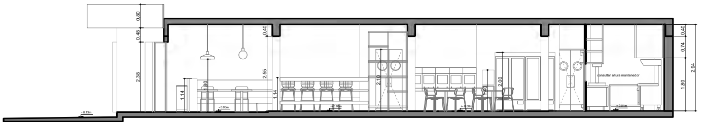
CORTE A-A
