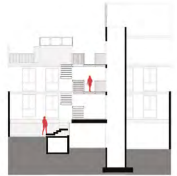
CORTE B-B ESC. 1:50
