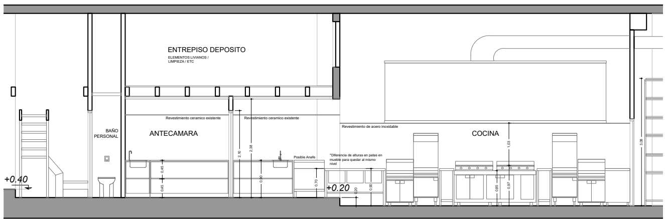
ELEVACIÓN COCINA - ESC. 1:50
