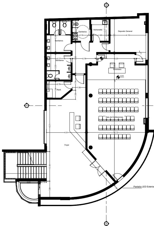
PLANTA TERCER PISO
