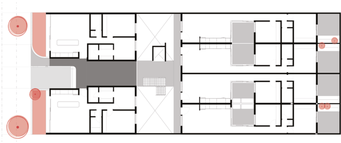
PLANTA BAJA ESC. 1:50
