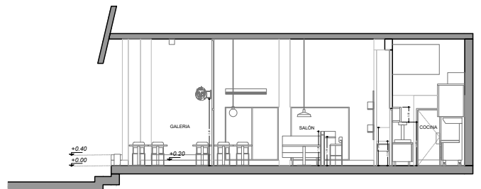
CORTE C-C
