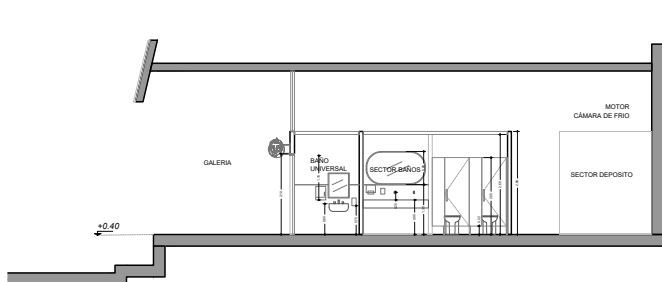
CORTE B-B
