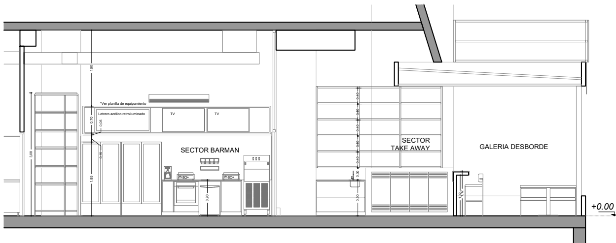
ELEVACIÓN BARRA INTERIOR Y EXTERIOR - ESC. 1:50
