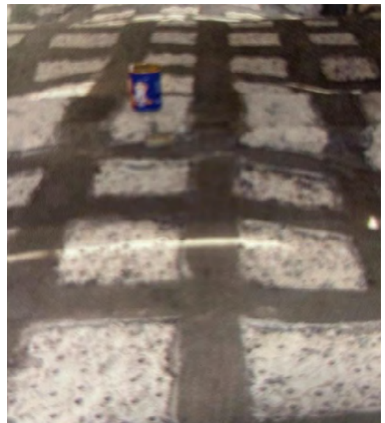
Refuerzo estructural con fibra de carbono.
