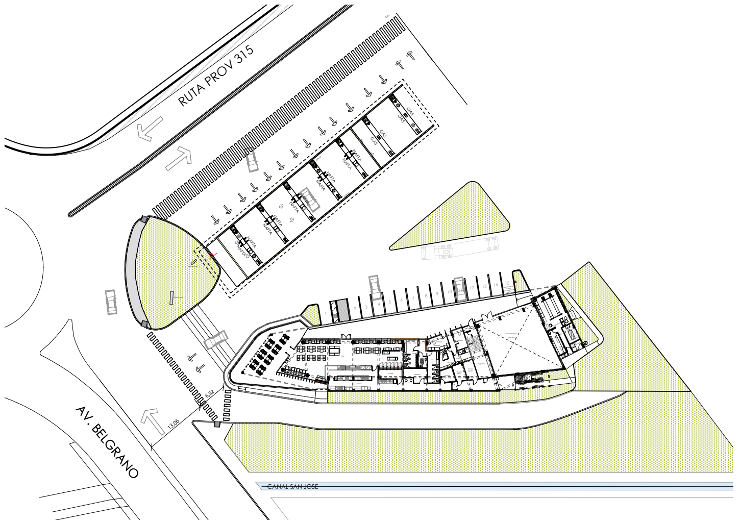
PLANO DE CONJUNTO
