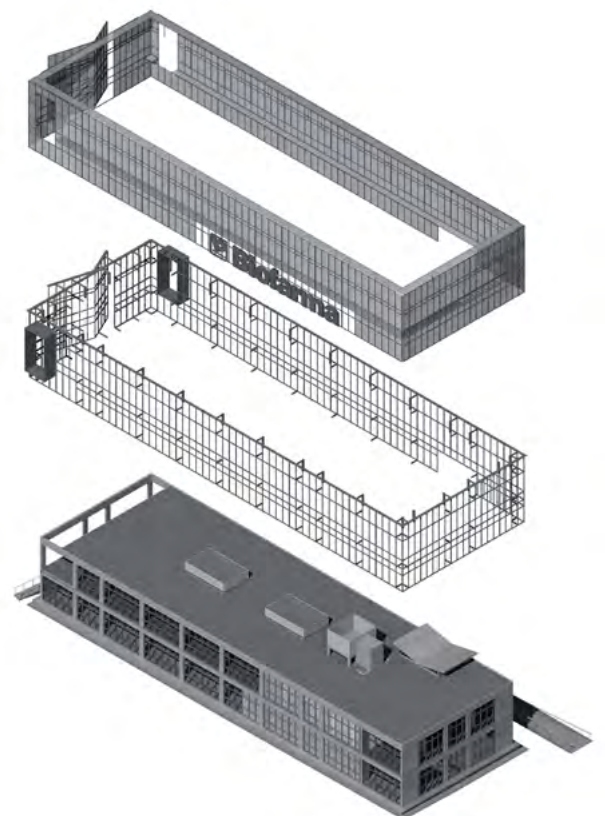
DESPIECE AXONOMÉTRICO ESC. GRÁFICA
