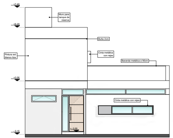
VISTA FRENTE
