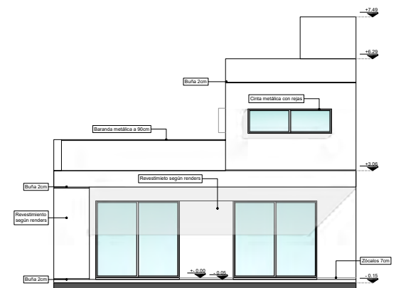
VISTA CONTRAFRENTE
