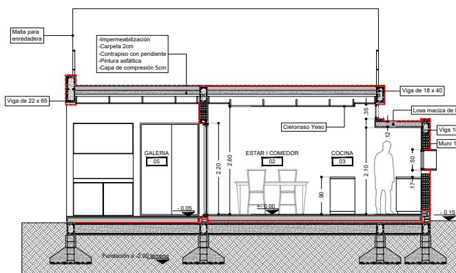
CORTE B - B
